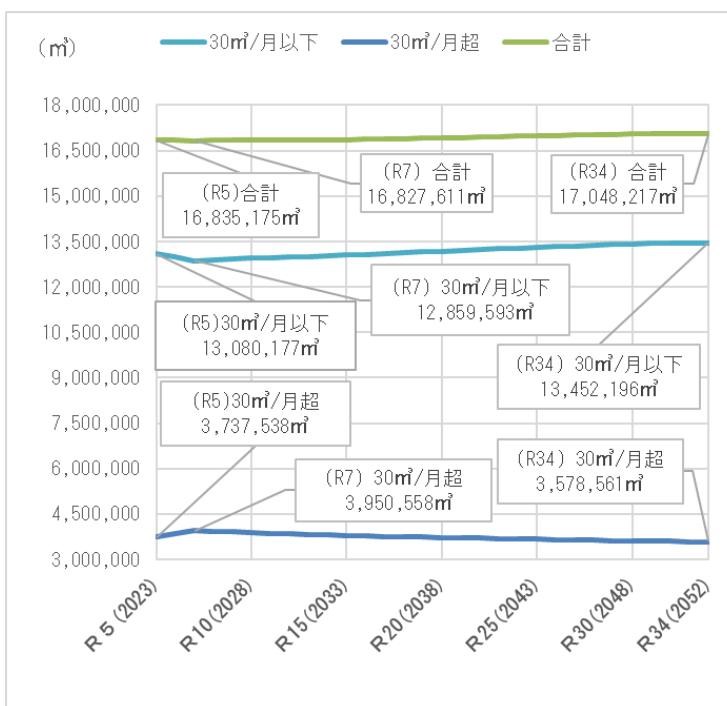
図表 4-2 有収水量の予測
