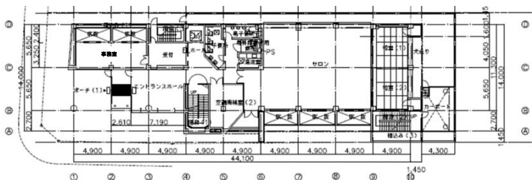
1階 平面図
