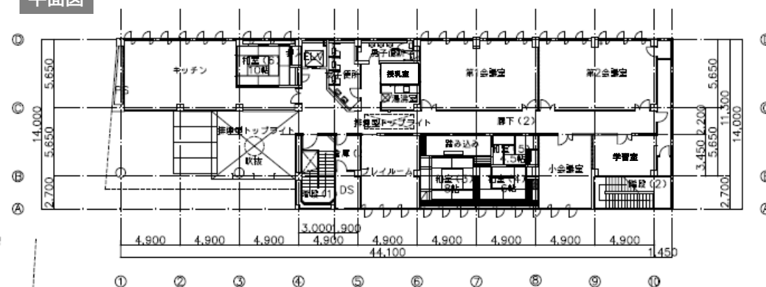
2階 平面図
