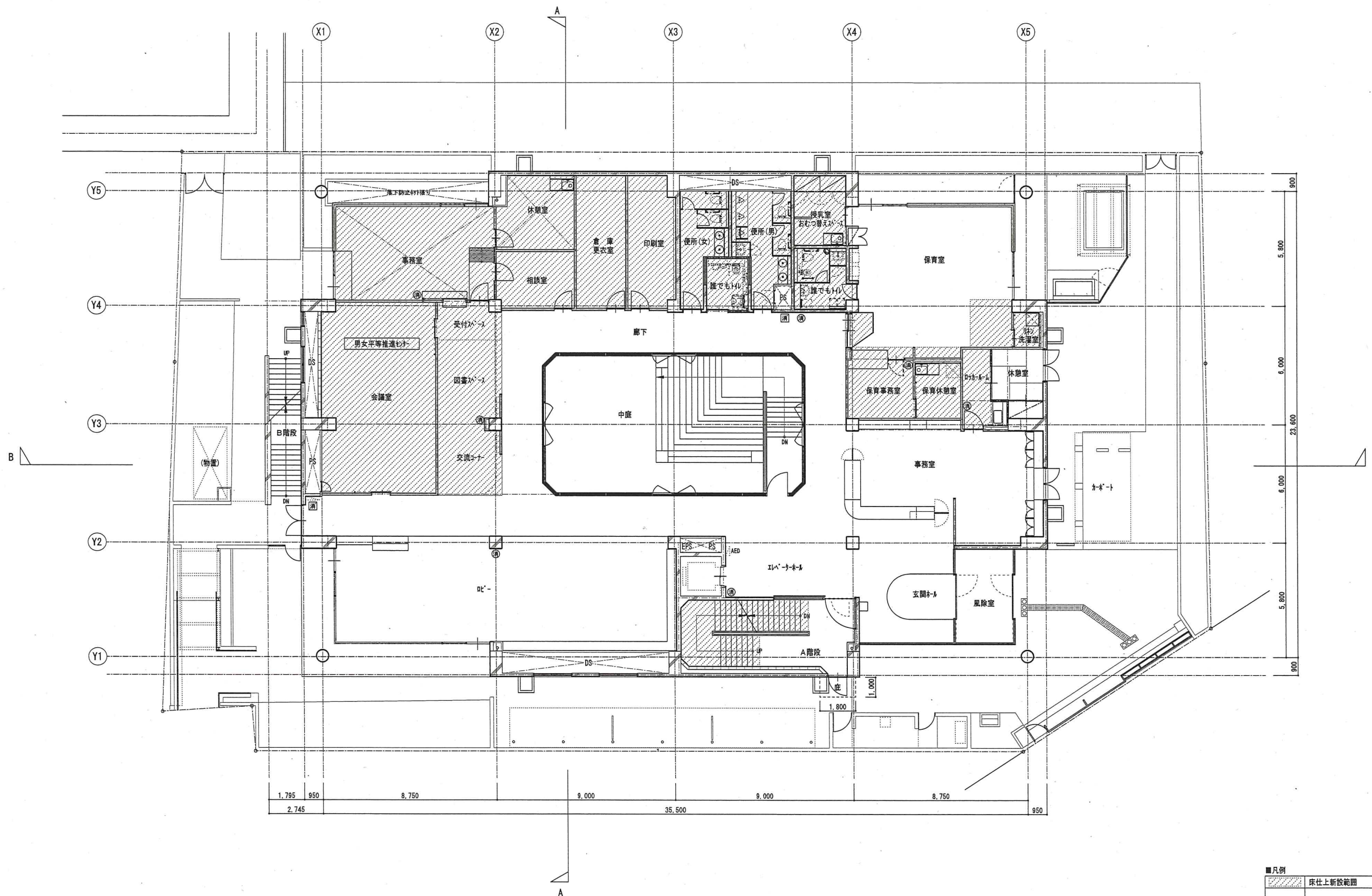
1階平面図
