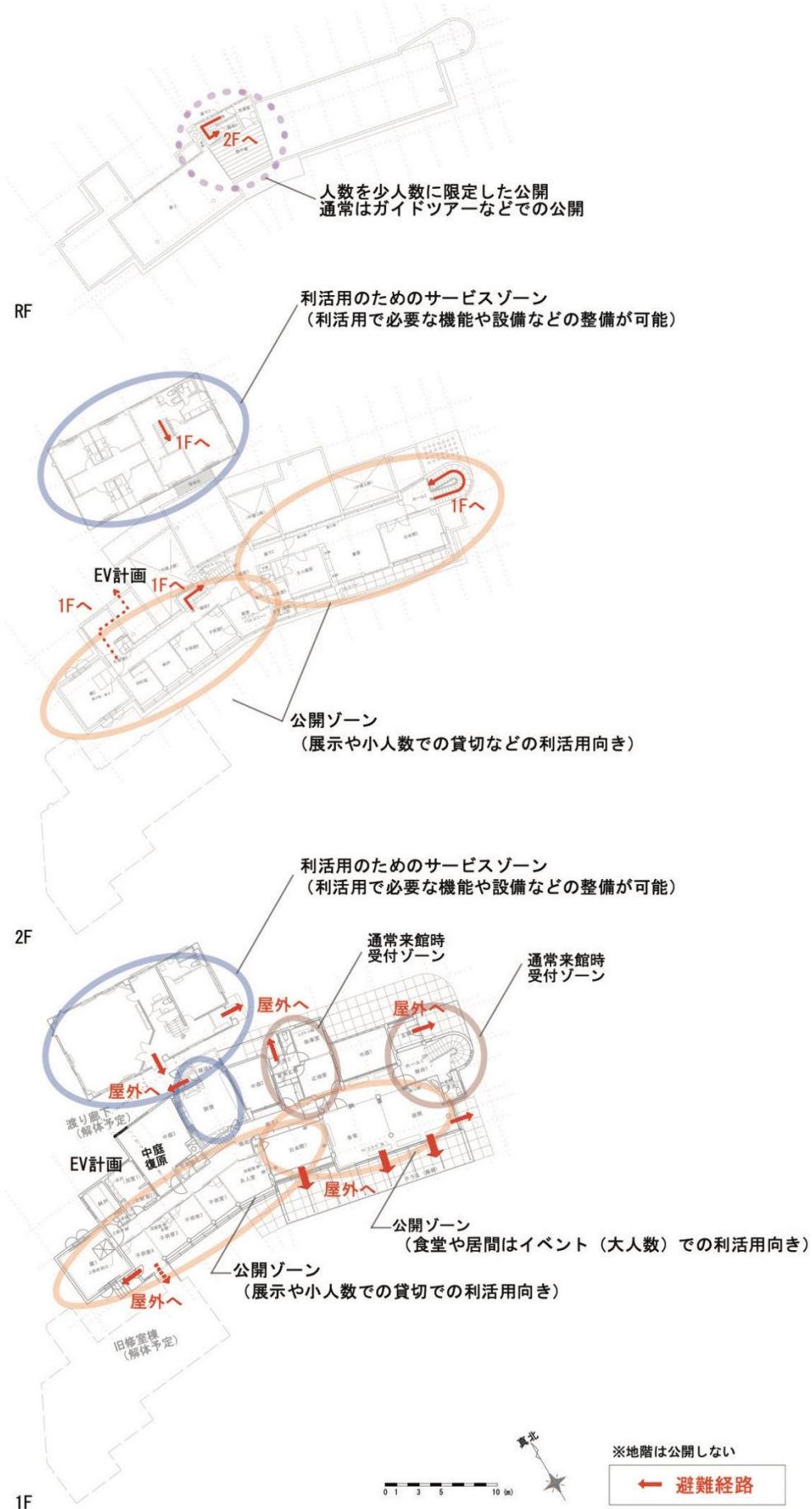
図 4-3 避難経路検討図
