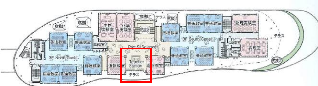
3階平面 (高等学校)
