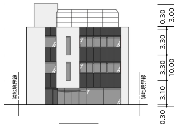
西立面図
