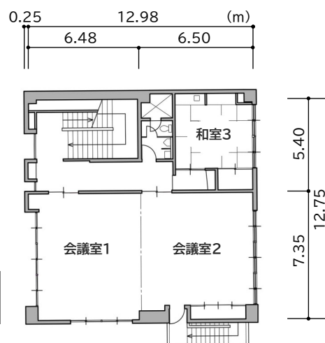
3階 平面図
