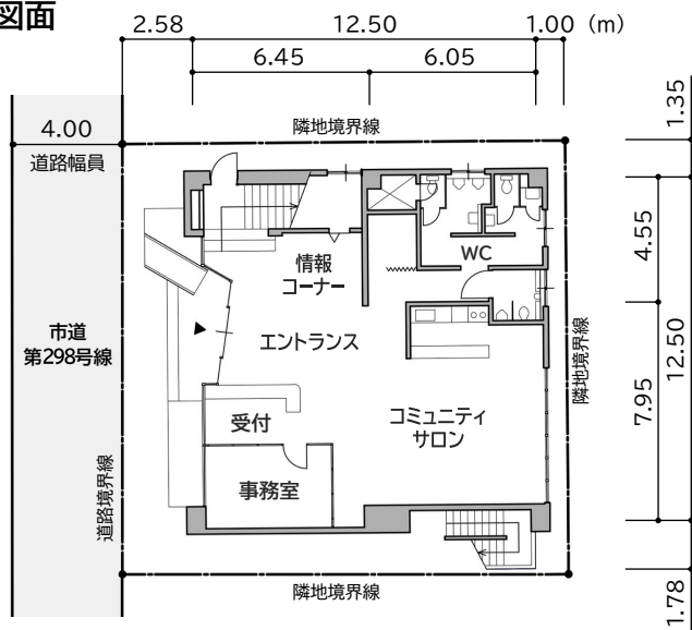
1階 平面図
