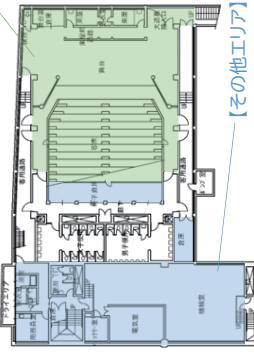
B1F平面図
