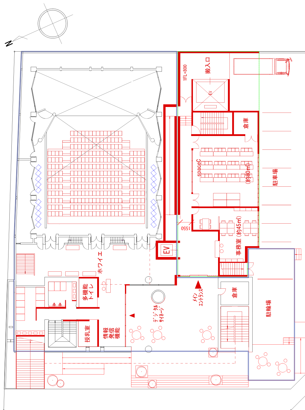
1 階平面図
