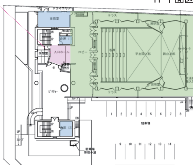
1F平面図
