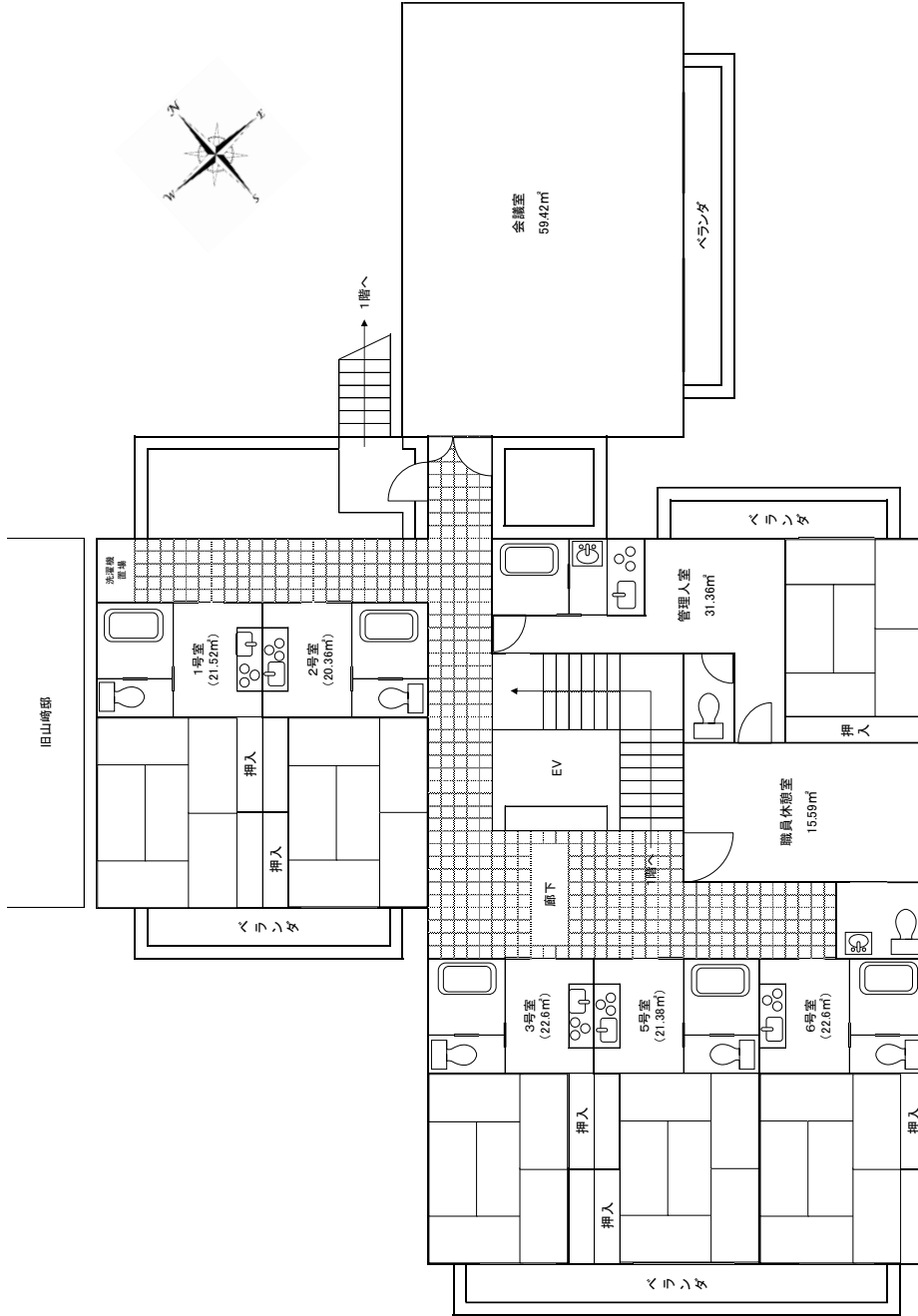
武威野市立北町高齢者センター本館2階平面図
