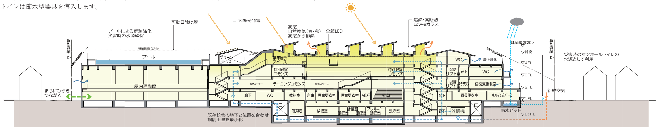
環境配慮イメージ図(長手断面)
