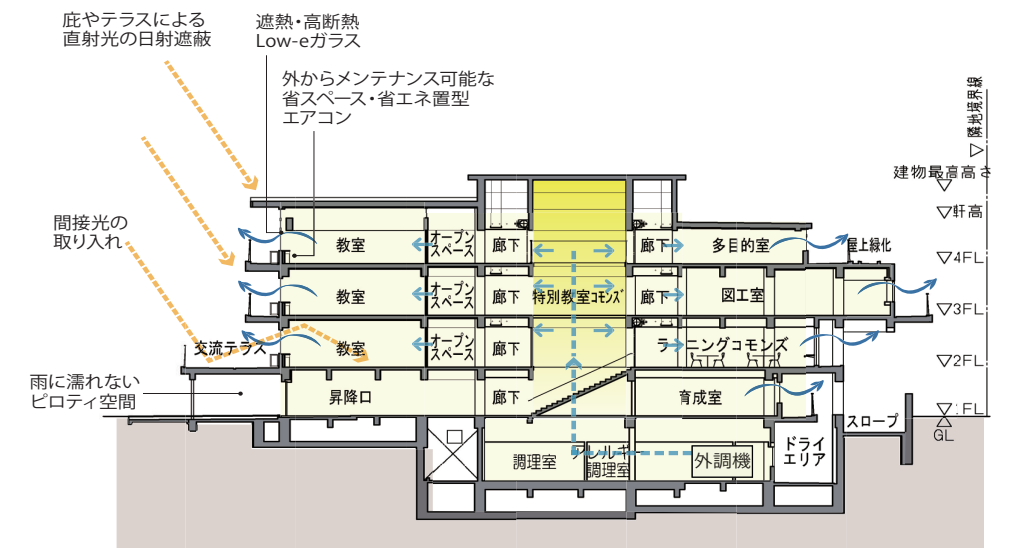
環境配慮イメージ図(短手断面)
