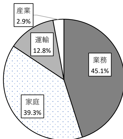
■図表6 武蔵野市のエネルギーの使用に伴う二酸化炭素の部門別構成
