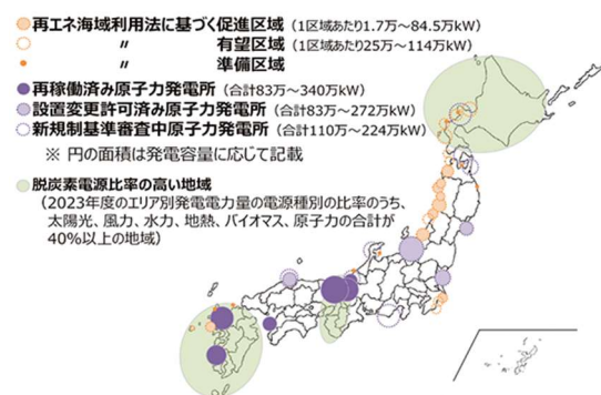
脱炭素電源の立地状況・規模 (出典:エネルギー白書2025)
