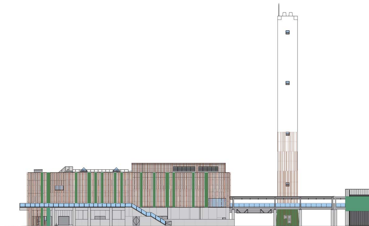
北立面図 (野球場側)
