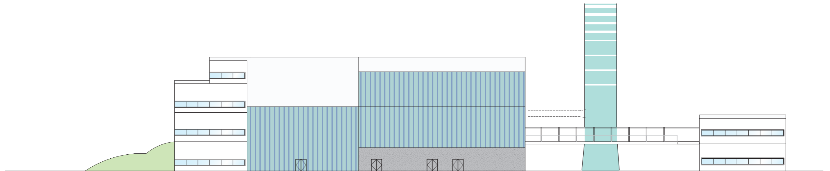
南側立面図
