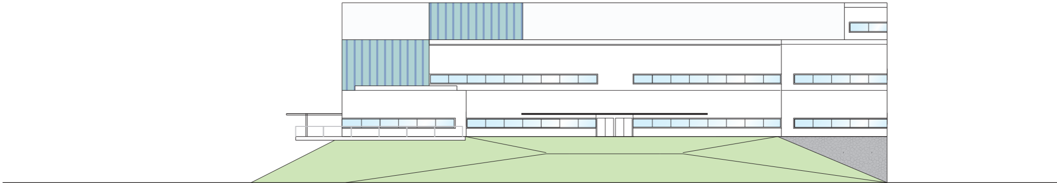
東側立面图
