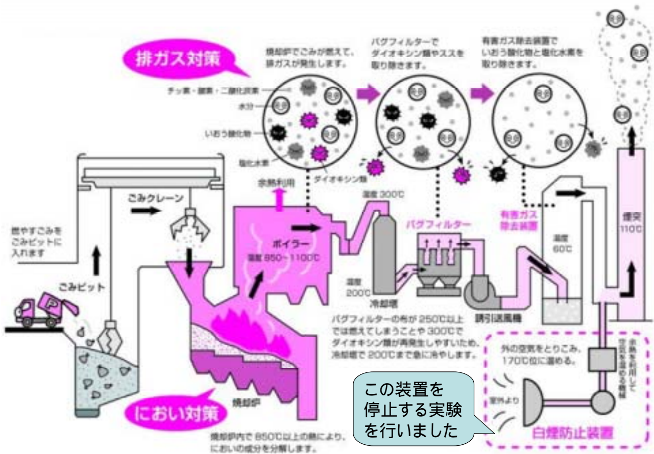
工場フロー図
