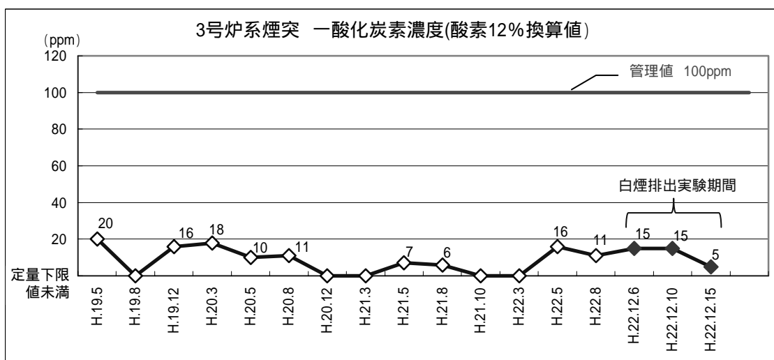
図-7 一酸化炭素濃度(酸素 12%換算値)の測定結果
