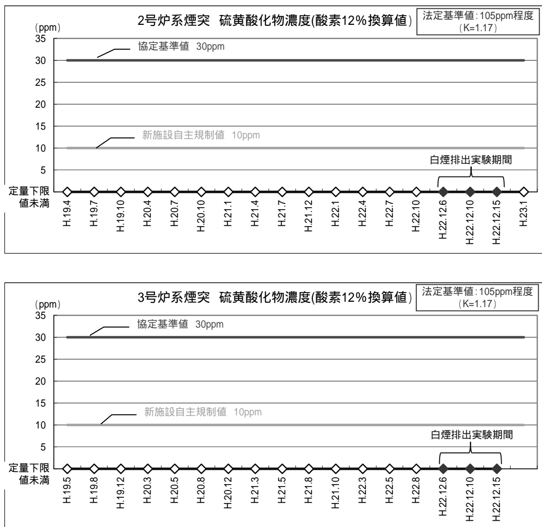
図-1 硫黄酸化物濃度(酸素 12%換算値)の測定結果
