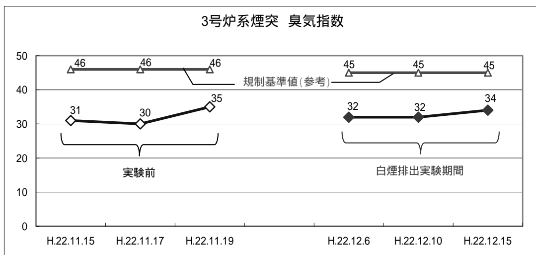
図-8 臭気指数の測定結果
