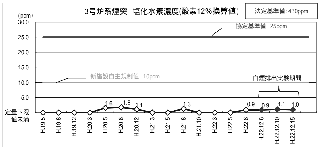
図-5 塩化水素濃度(酸素 12%換算値)の測定結果
