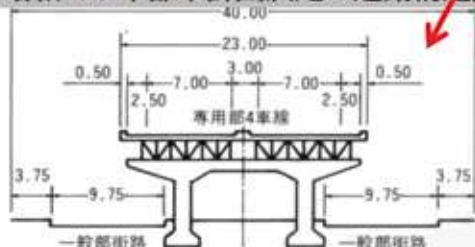
昭和 41 年都市計画決定の道路構造図
