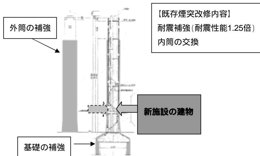
図 -1 既存煙突補強のイメージ
