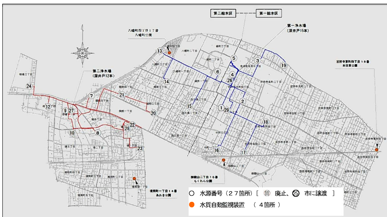
図 7 採水場所と給水区
