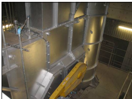
二次破碎機
