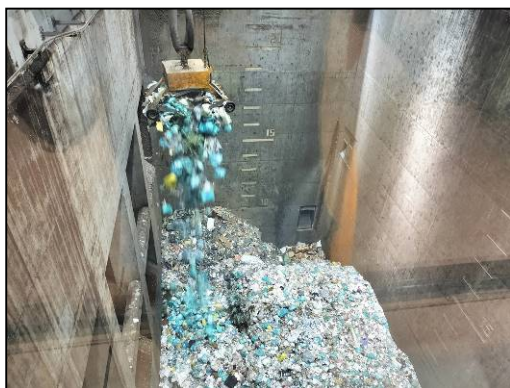
収集車がごみをおろす様子（上）、可燃ごみピットの様子（下）
