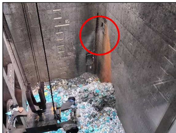
可燃ごみピットの落ち口
