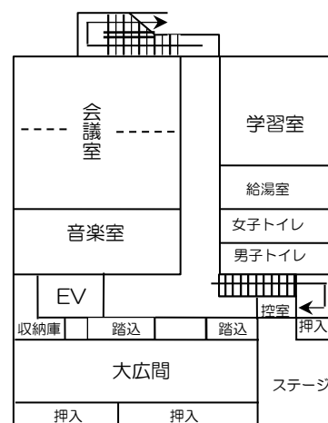
2 階平面図
