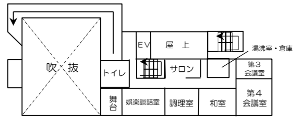
2階平面図
