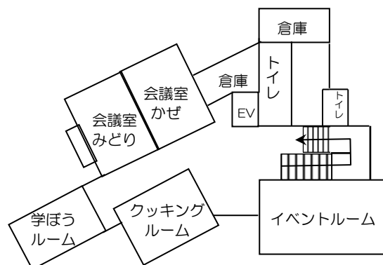
2 階平面図
