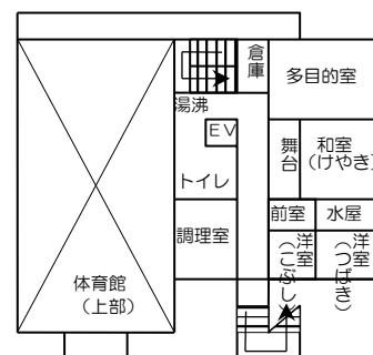
2階平面図
