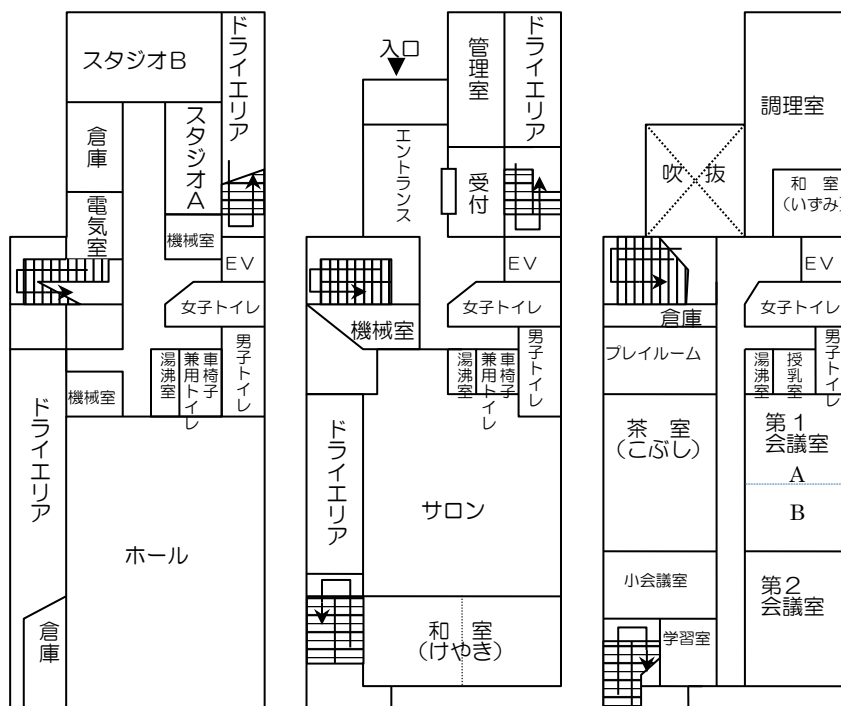
1階平面図
