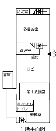
1階平面図
