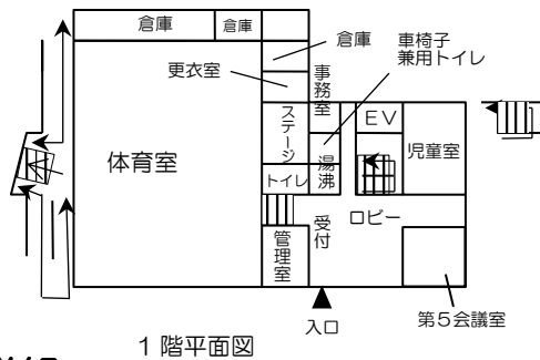
1階平面図
