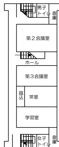
3階平面図
