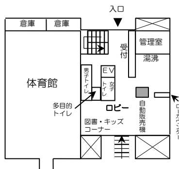
1階平面図
