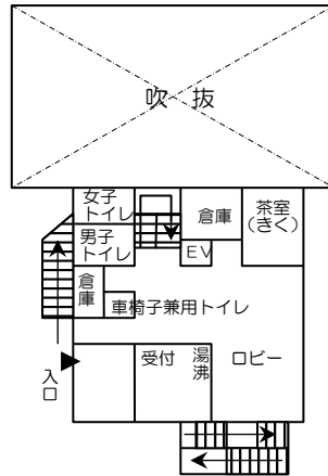
1階平面図
