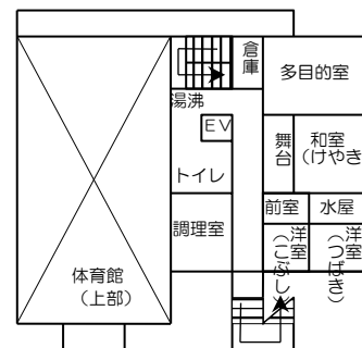
2階平面図
