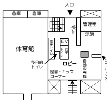
1階平面図
