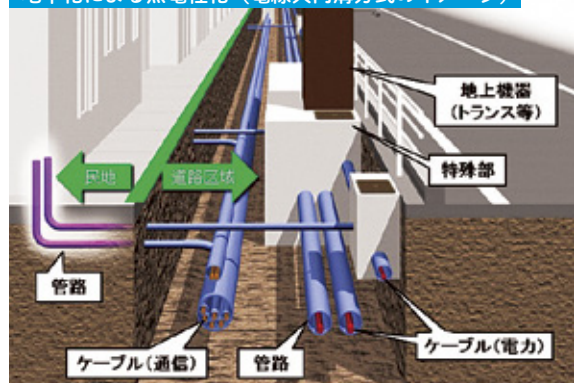
地中化による無電柱化（電線共同溝方式のイメージ）
