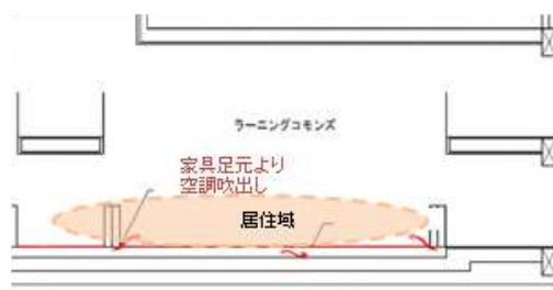
アンダーフロア空調とすることで、天井高を確保します
