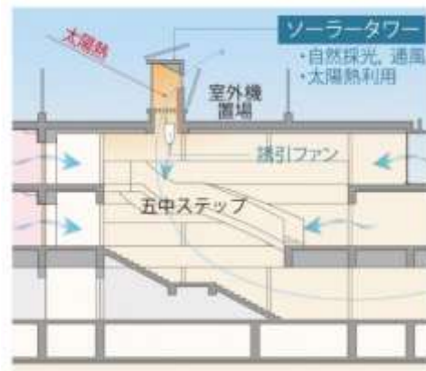
ソーラータワーイメージ (五中ステップ断面)
