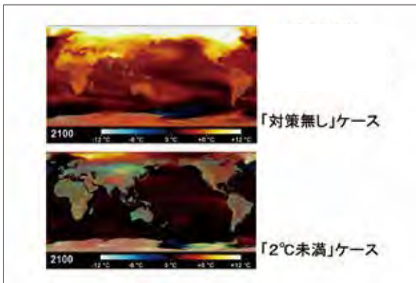
気温変化シミュレーション MIROC5気候モデルによる(AORI/NIES/JAMSTEC/MEXT)
