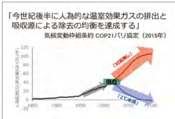
「2℃未満」目標を達成する排出削減経路
