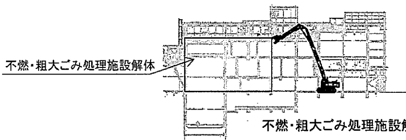
段階解体図(1)
