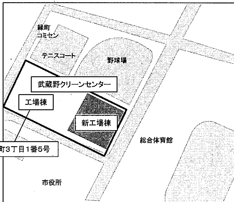
配置図・解体工事範囲図
